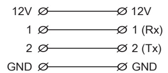
Elektrisch schema
