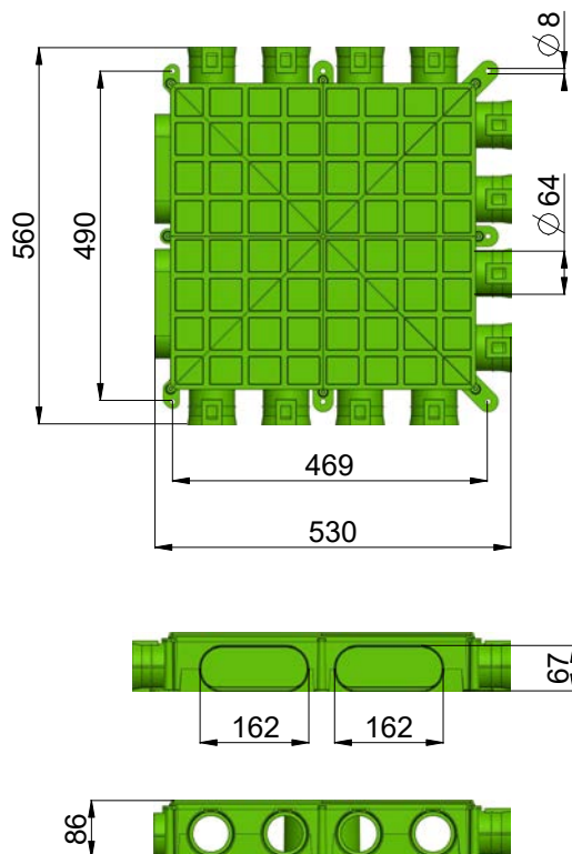
Caractéristiques de pulsion et d'extraction
